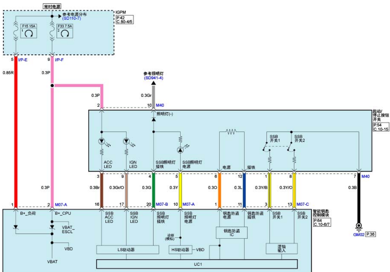
智能钥匙模块系统(3)
